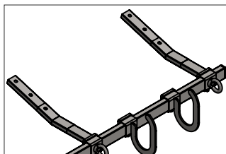
Balestra regolabile di ancoraggio su superficie inclinata
