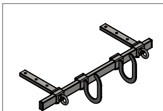
Balestra regolabile di ancoraggio su superficie dritta e/o piana
