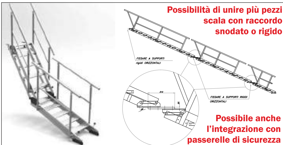
In esempio disegno articolo SCA AV60-80/14
