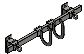
Balestra regolabile di ancoraggio a muro o su parete verticale
