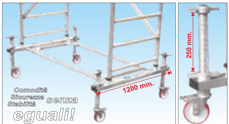
In foto configurazione completa art. ITAL-03 BL
