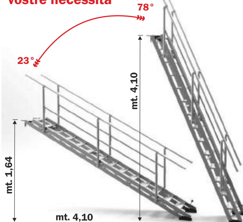
In esempio disegno articolo SCA AV60-80/14
