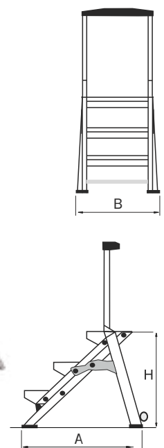
In foto articolo SCA WT/03
