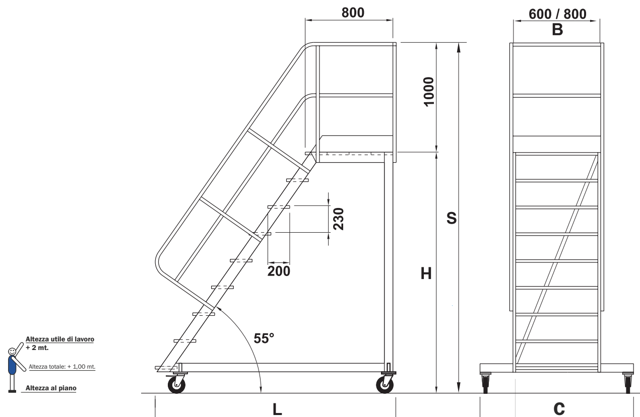
Gradino piano profondo 200 mm.
