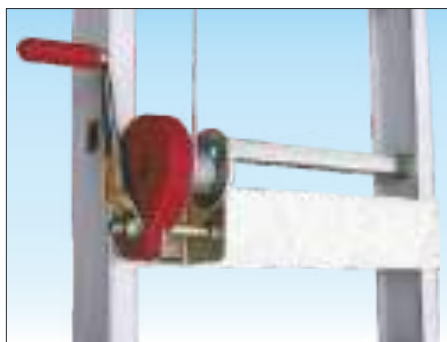
Argano professionale con frizione in salita e discesa
