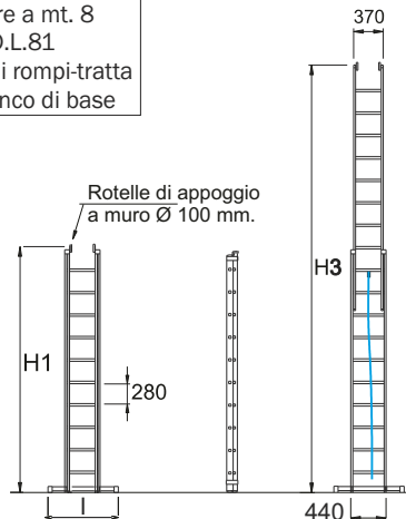
In foto articolo SCA 3051N/18
