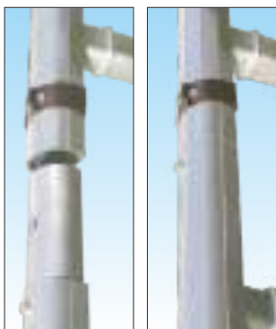
Innesto dei montanti verticali in profilo di alluminio con bloccaggio automatico ad elevata tenuta
